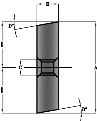
Lame a 2 fili
