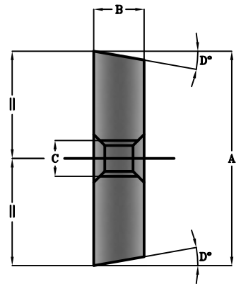
Lame a 2 fili complanari
