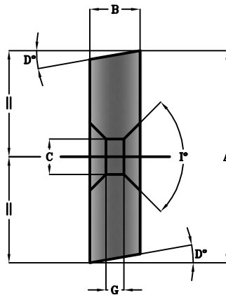
Lame a 2 fili fori svasati
